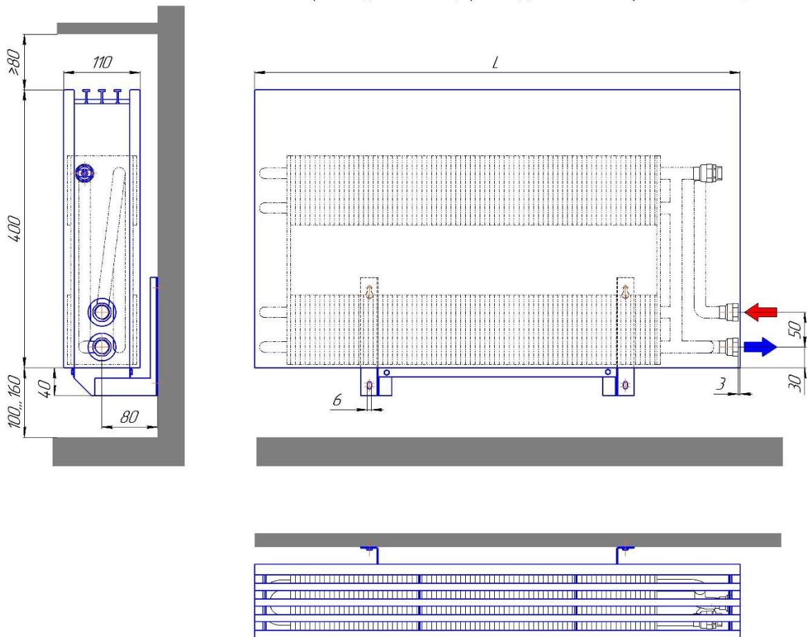
Монтажная схема настенного конвектора "Элегант 110x400 4то бок Стен" с боковым присоединением (присоединительная резьба - 1/2")
