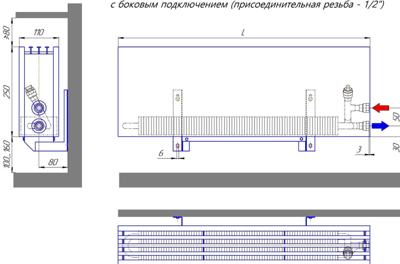
Монтажная схема настенного конвектора "Элегант 110x250-2то бок Стен" с боковым подключением (присоединительная резьба - 1/2")
